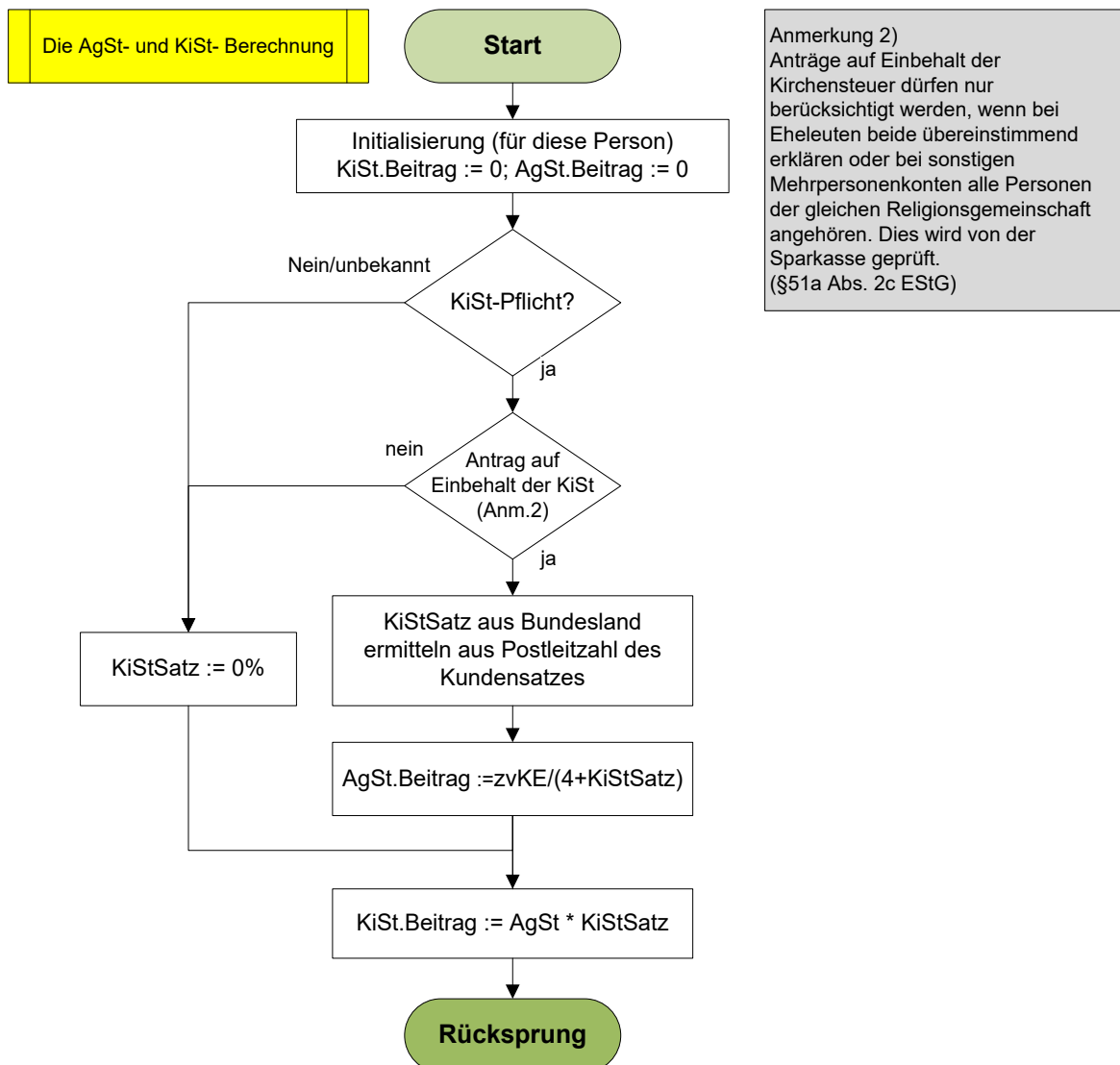
Abbildung 301: Ablaufplan Steuerrechnung: Unterroutine AGSt und KiSt
