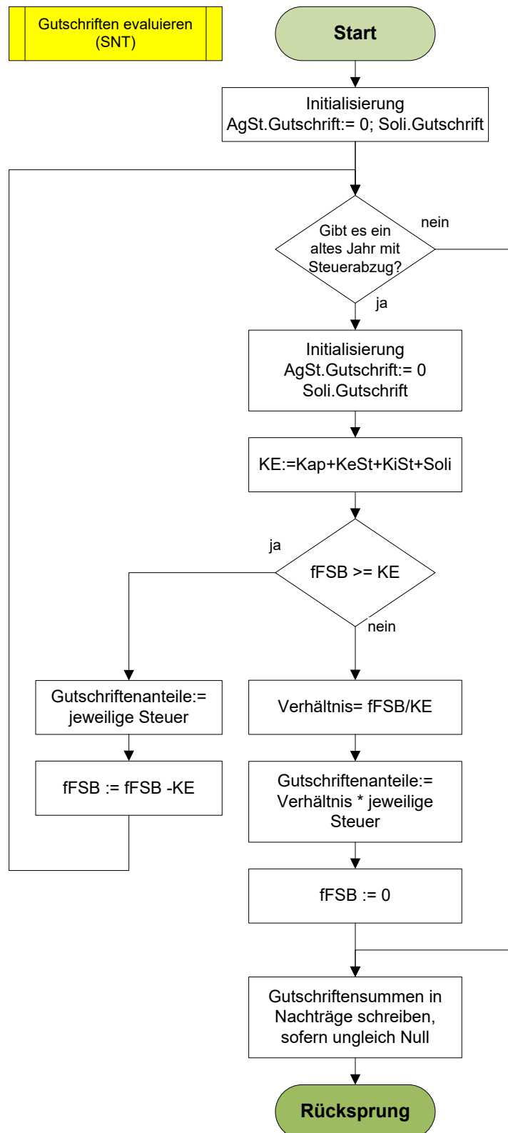
Abbildung 302: Ablaufplan Steuerrechnung: Unterroutine Gutschriften
