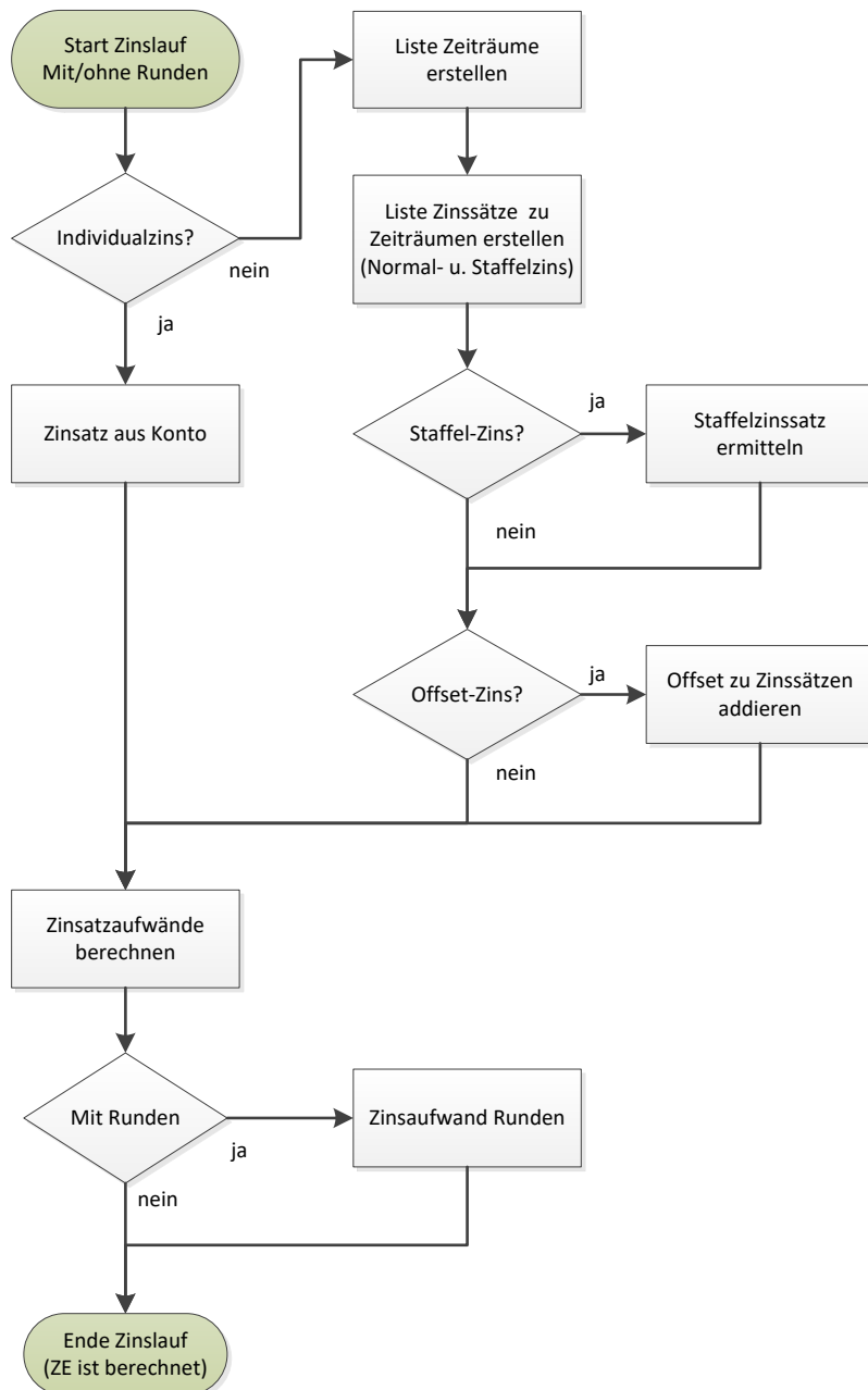
Abbildung 299: Ablaufplan Zinsrechnung (Unterroutine)
